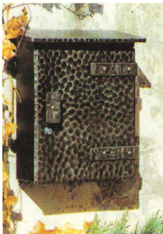
52/2 Briefkasten „Royal“ , superschwer, verz. Stahlblech, geschmiedet m. gehämmelter Vorderfront, Maße 36x32x10 cm
