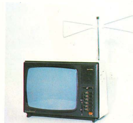
Nordmende Portable-Fernseh er Portino, 31-cm-Rechteck-Bild- schirm, volltransistorisiert, 6 Programmtasten mit elektroni- scher Abst., für Netz und Batta- riebetrieb
